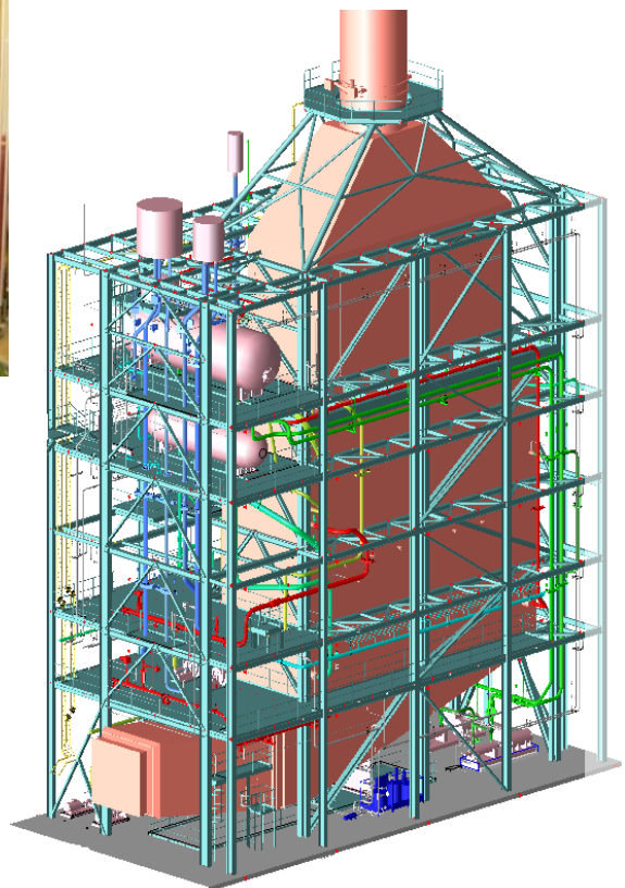
3D model of HRSG
